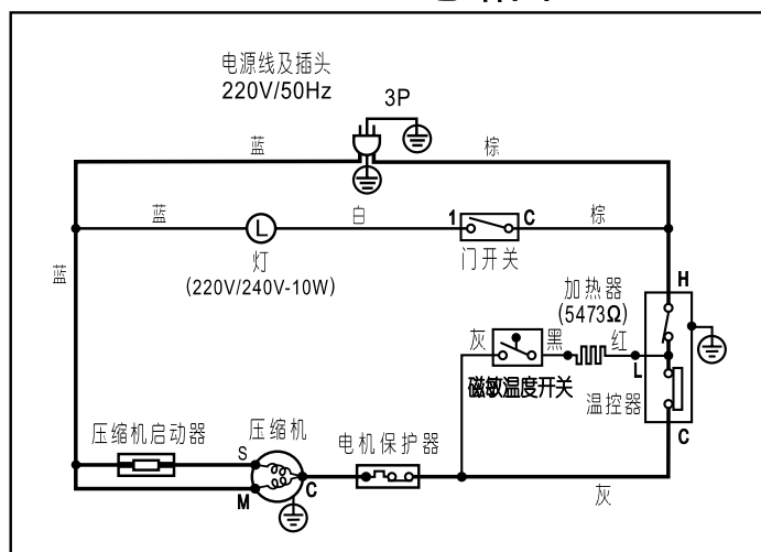
NR-B23S7电路图
